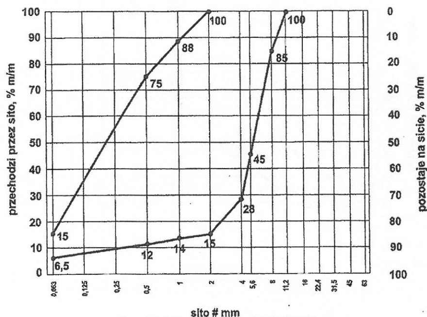
Rys. 1.5. Uziarnienie mieszanki CBGM 0/8
